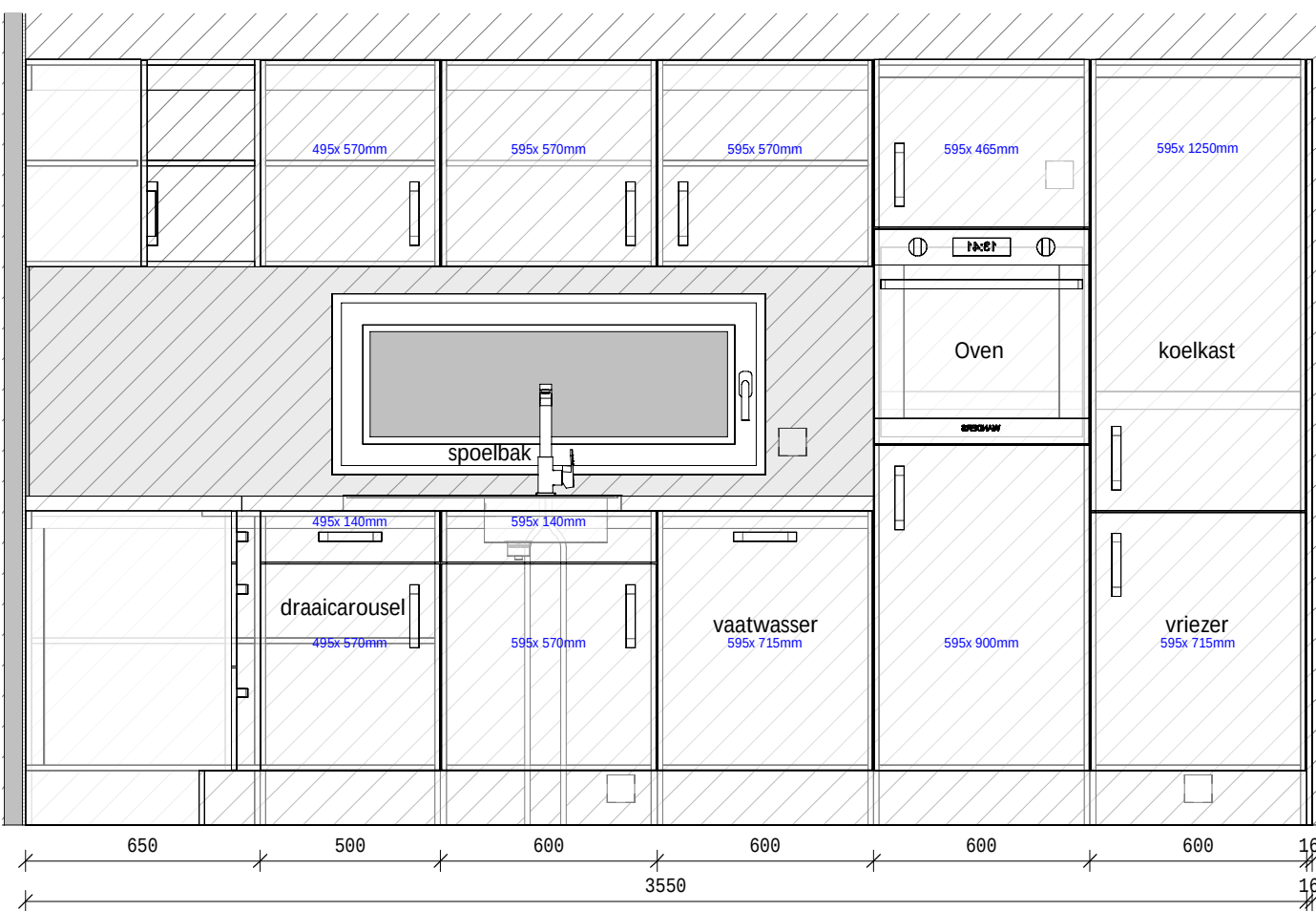
P- Keuken aanzicht 1 schaal: 1 : 20
