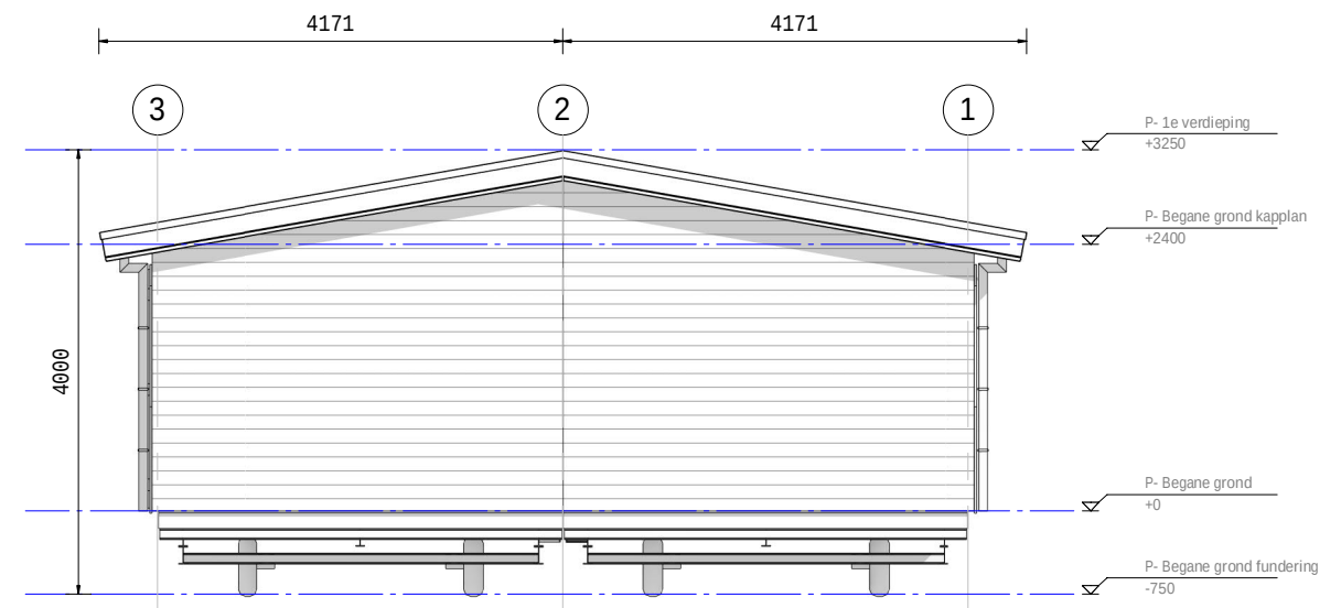
RECHTERZIJGEVEL
