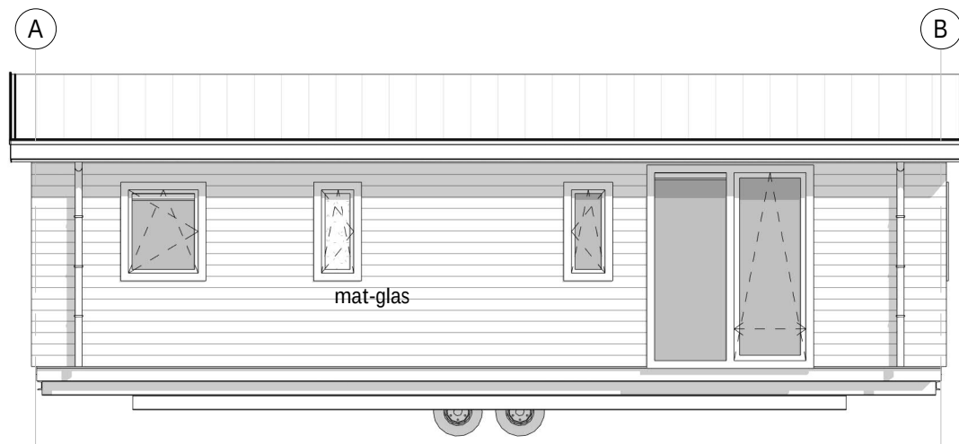
ACHTERGEVEL
