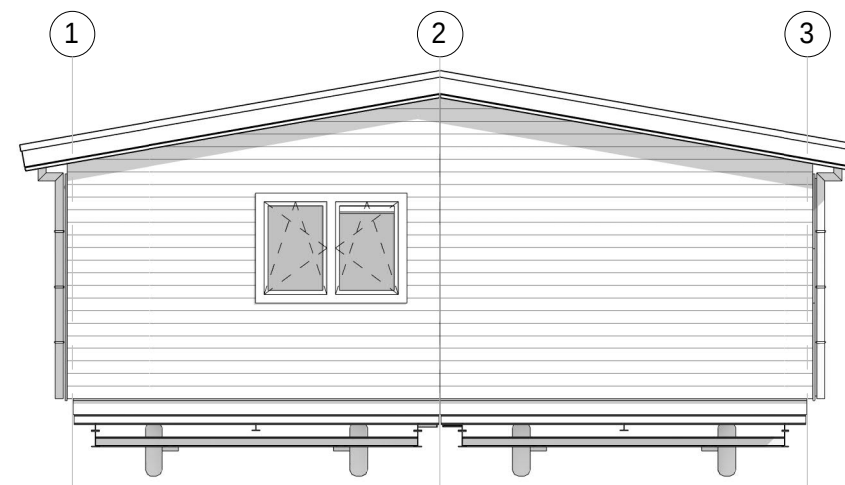
LINKERZIJGEVEL
